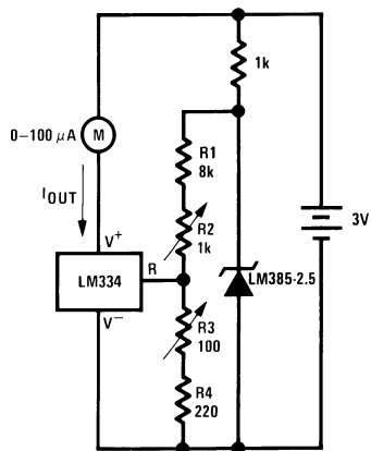
0°C–100°C Thermomemter
