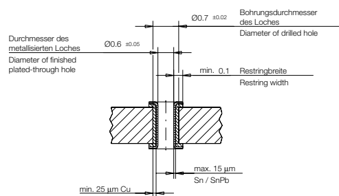
Schichtaufbau im metallisierten Loch für EE-Kontakt Metal plating of plated-through hole for EE-contact
