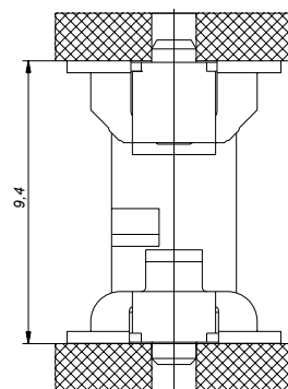
Federleiste niedere Bauform
