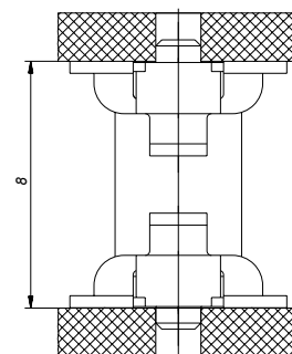
Federleiste niedere Bauform
