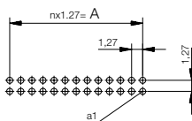
Lochbild für Leiterplatte Board hole pattern
