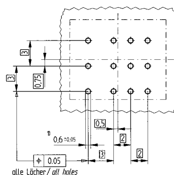
Lochbild für Leiterplatte / Board hole pattern
