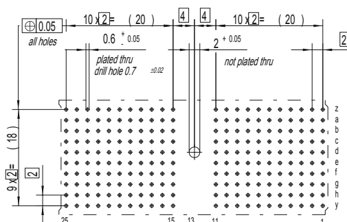
Lochbild fuer Leiterplatte (Besteckungsseite)
