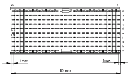
Lochbild fuer Leiterplatte (Bestueckungsselle)
