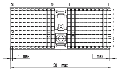
Lochbild fuer Leiterplatte (Besteckungsseite)
