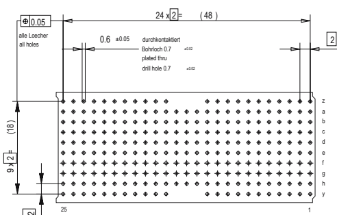
Lochbild fuer Leiterplatte (Bestueckungsselle)
